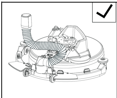
3 После очистки установить шланг в исходное положение.
